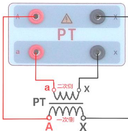
图 24 , PT 变比极性接线图
