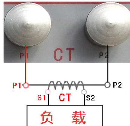
图 17、CT 一次通流接线图
