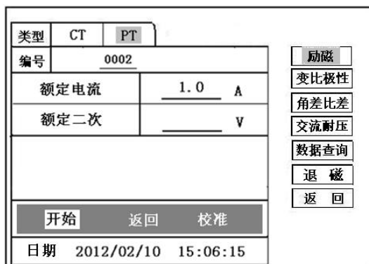
图 20，PT 励磁特性参数设置界面
