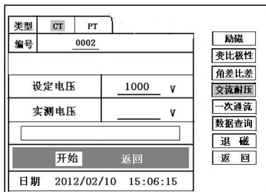
图 18、CT 交流耐压测试界面
