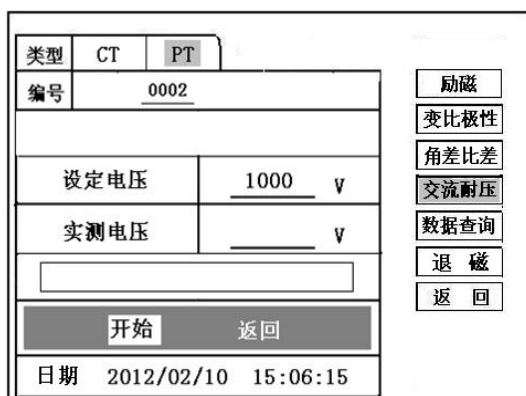
图 27, PT 交流耐压测试界面
