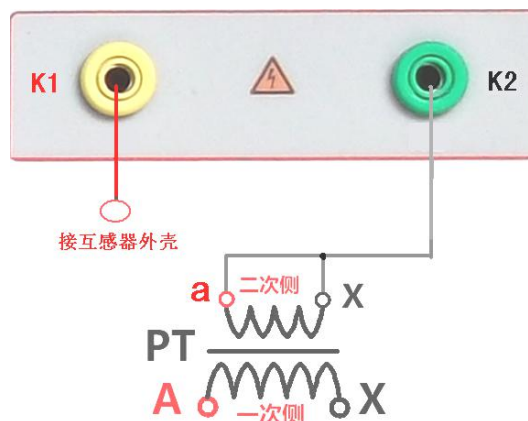
图 28, PT 交流耐压接线图
