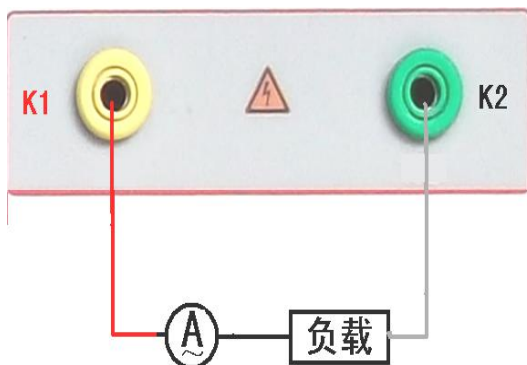
图 34, 电流校准接线图
