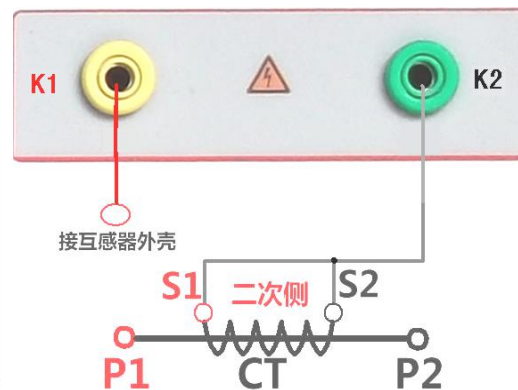
图 19、CT 交流耐压接线图
