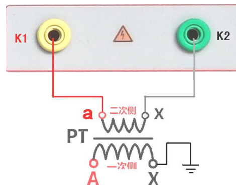
图 21，PT 励磁特性接线图
