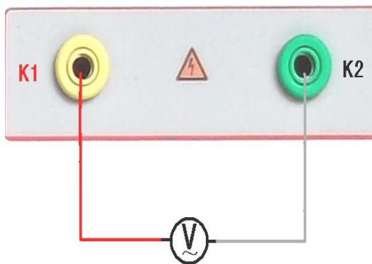
图 33, 电压校准接线图
