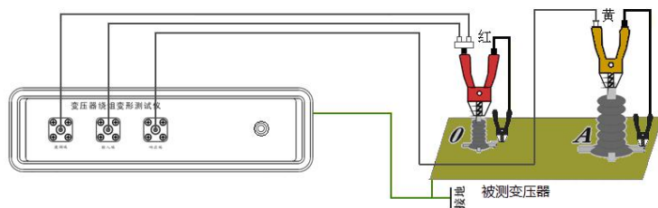
图2 接线示意图
