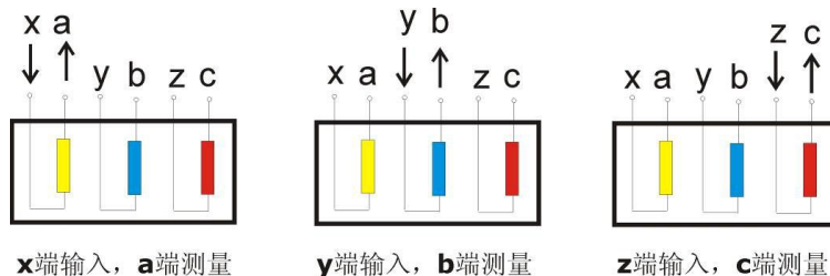
图6 外连接Δ接线
