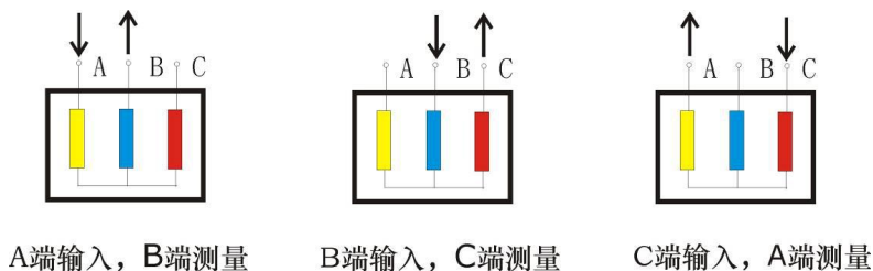
图4 Y 接线
