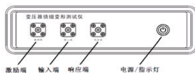
图 1a 变压器绕组变形测试仪前面板图(前面板)
