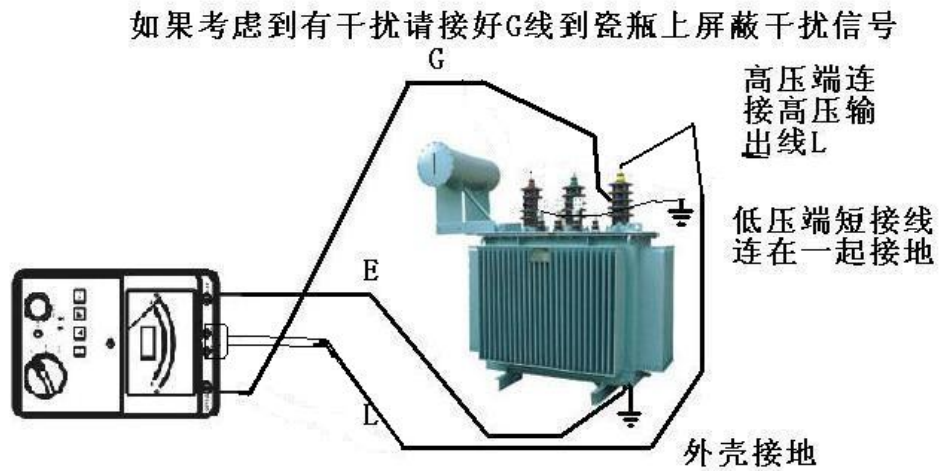
变压器高压端对地绝缘 (由此图示变化可测高低压端绝缘、低压端对地绝缘等)
