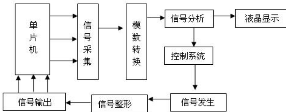
信号发生器原理图
