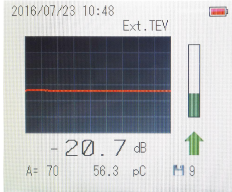
图六 TEV 模式测量界面
