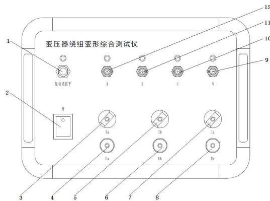
图 1 变压器绕组变形综合测试仪面板图
