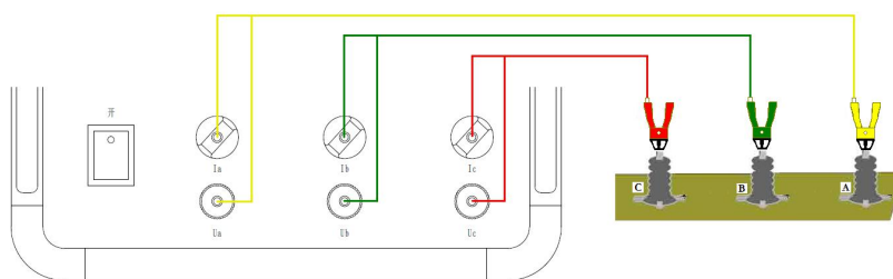
图 4 阻抗法接线
