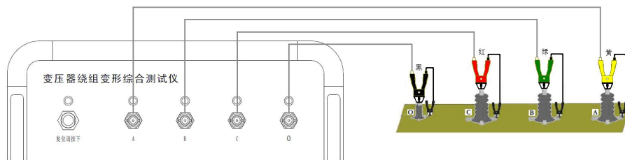
图 2 频响法测试接线图
