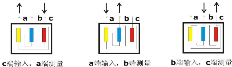
图 5 内连接 Δ 接线
