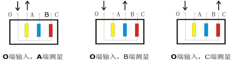
图 3 YN 接线
