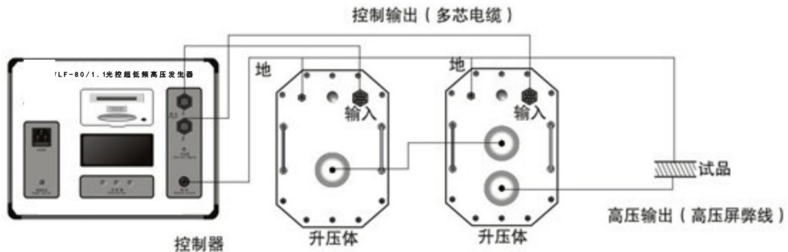
图 4b DYLF-V-90/1.1 (连线图)
