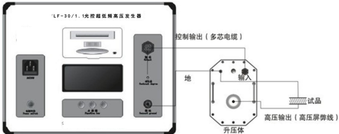
图 4a DYLF-V-40/1.1 或 DYLF-V-50/1.1 (连接图)
