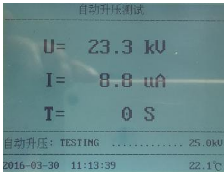
图 20 自动耐压试验升压界面
