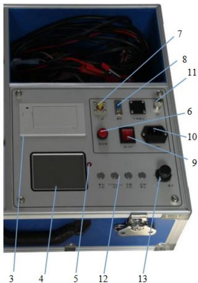
图 1 面板说明图
